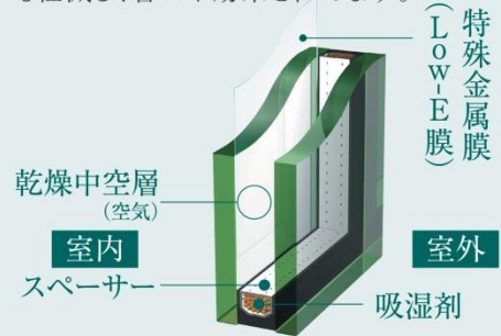
※Low-E複層ガラス概念図
